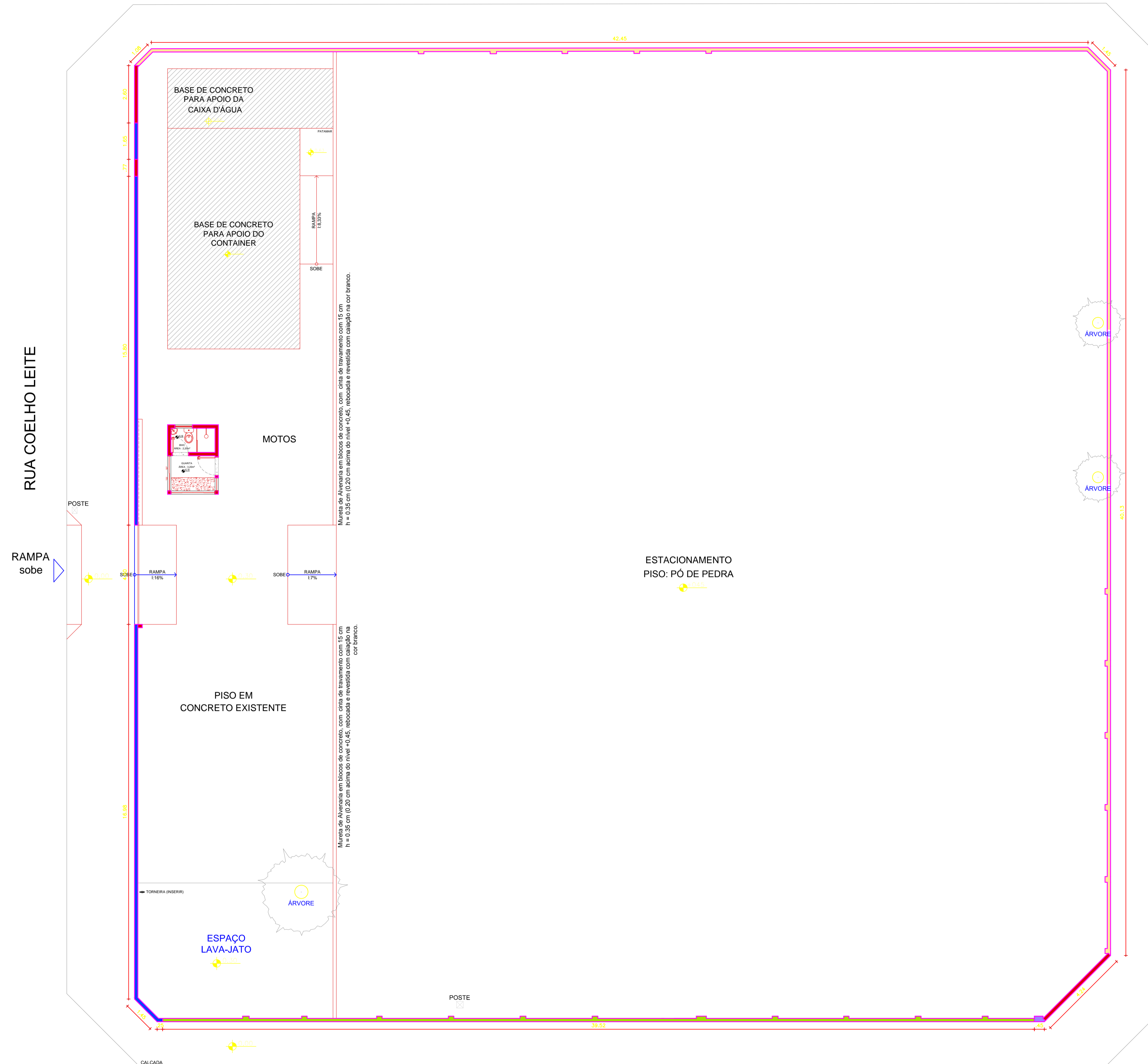
PLANTA DE REFORMA (MUROS) - ESTACIONAMENTO CASARÃO ESCALA: 1/200
