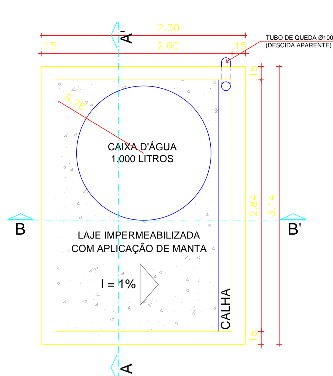
PLANTA DE COBERTA - GUARITA Esc.: 1/50
