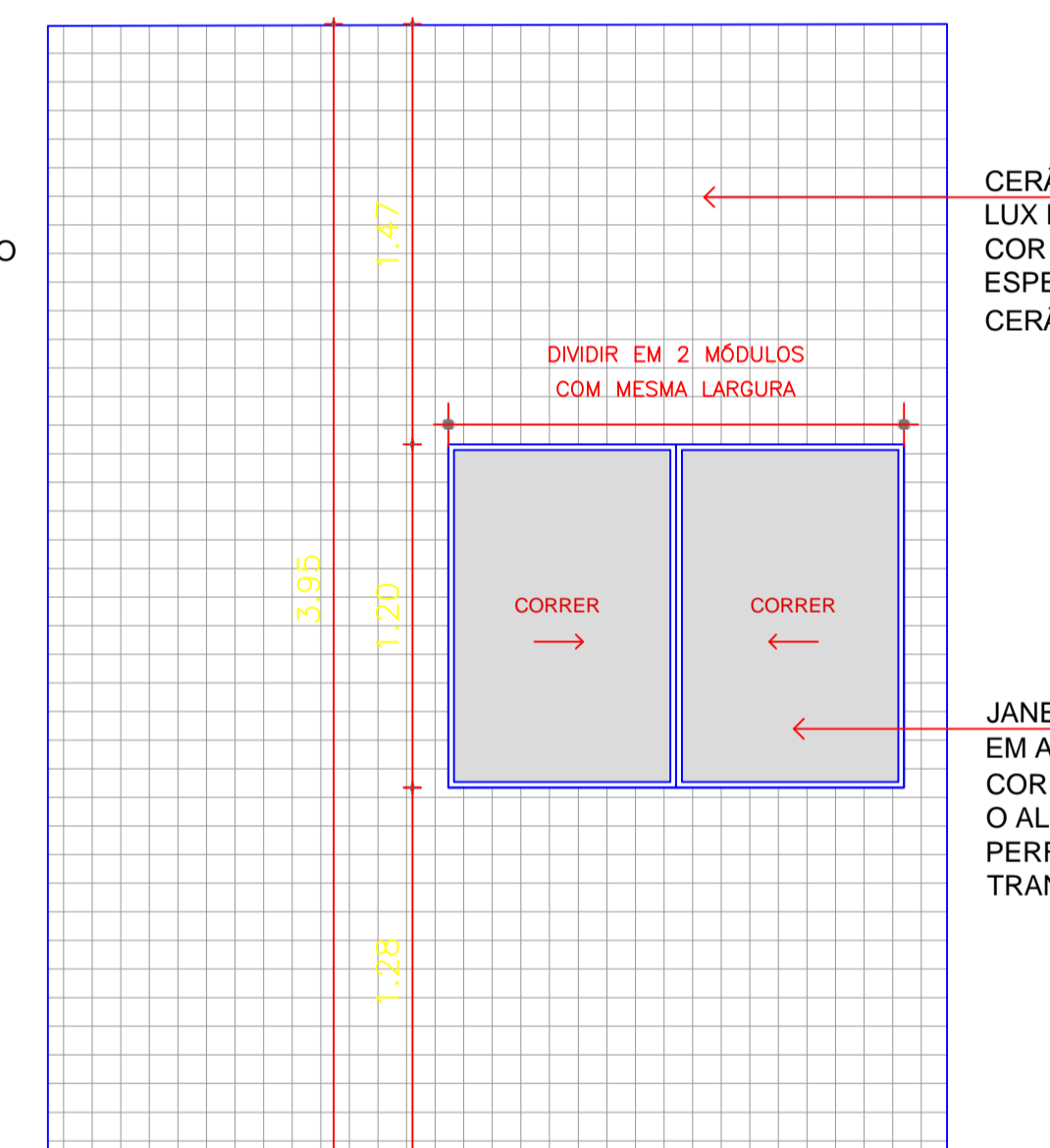
ELEVAÇÃO - VISTA 02 Esc.: 1/50
