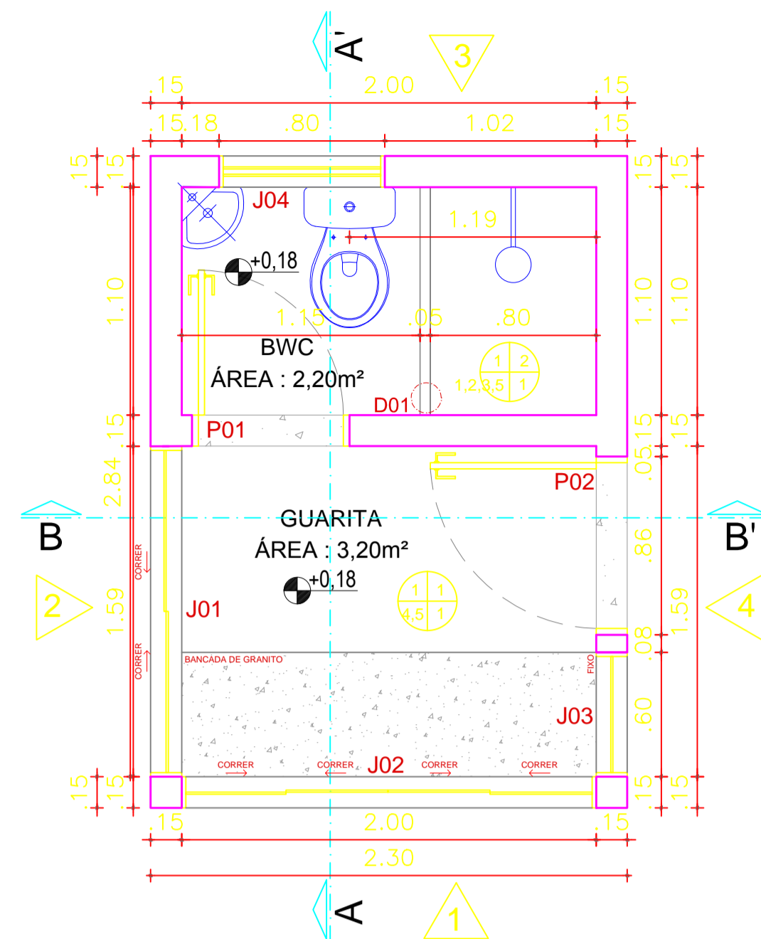
PLANTA BAIXA - GUARITA Esc.: 1/50
