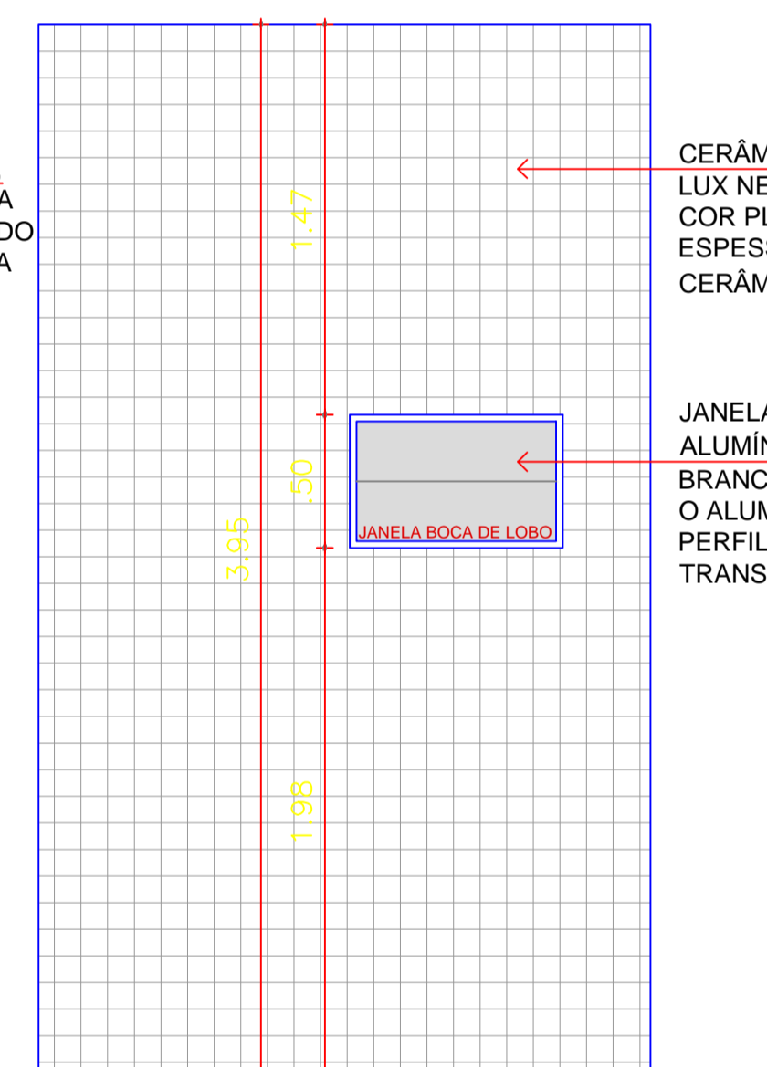
ELEVAÇÃO - VISTA 03 Esc.: 1/50
