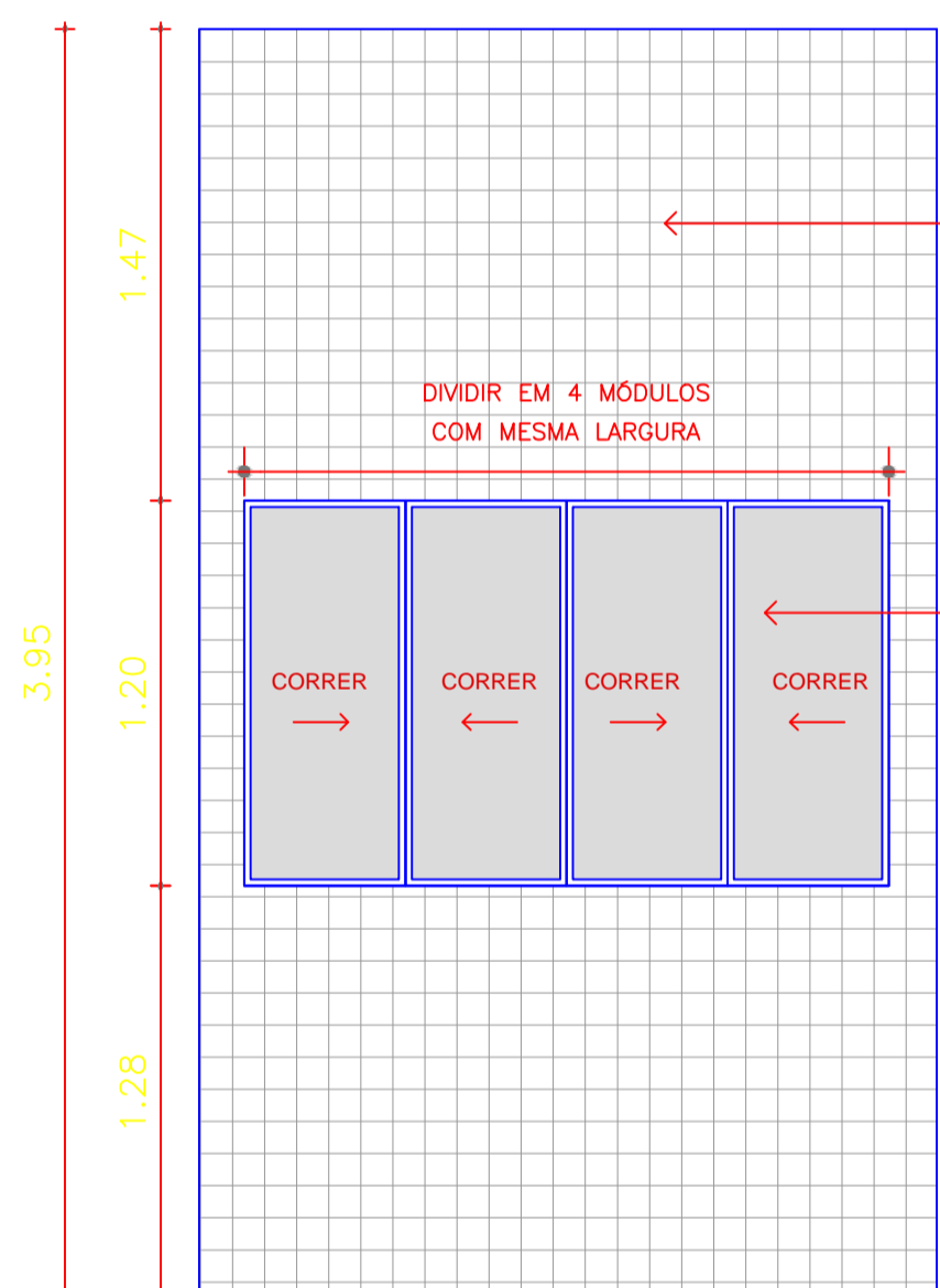
ELEVAÇÃO - VISTA 01 Esc.: 1/50
