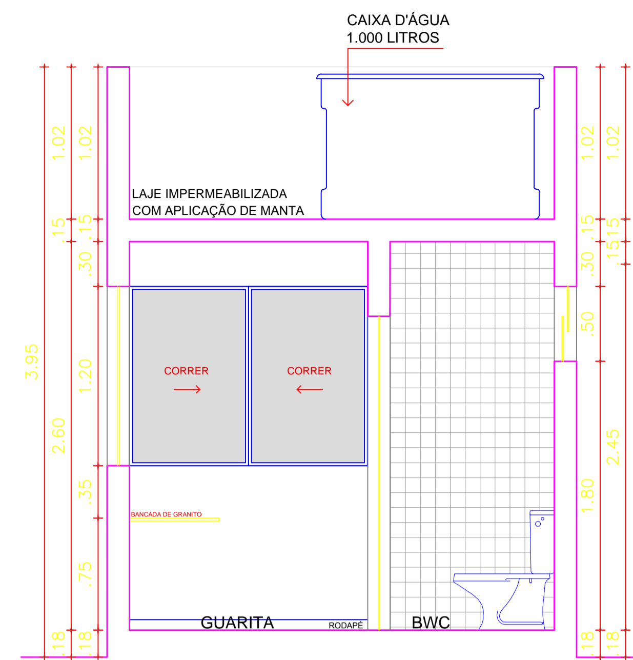
CORTE AA' Esc.: 1/50
