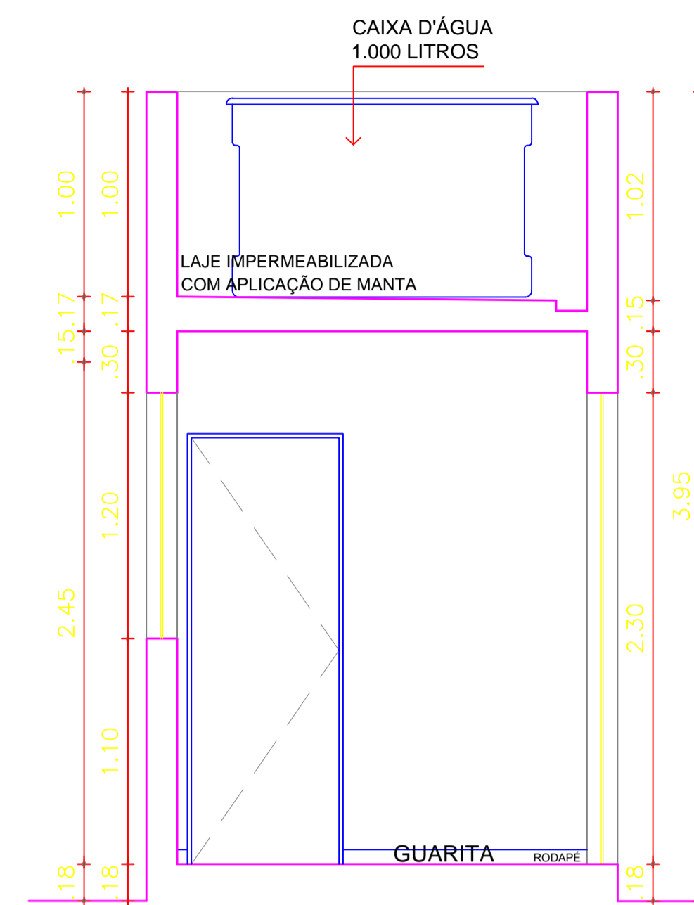
CORTE BB' Esc.: 1/50
