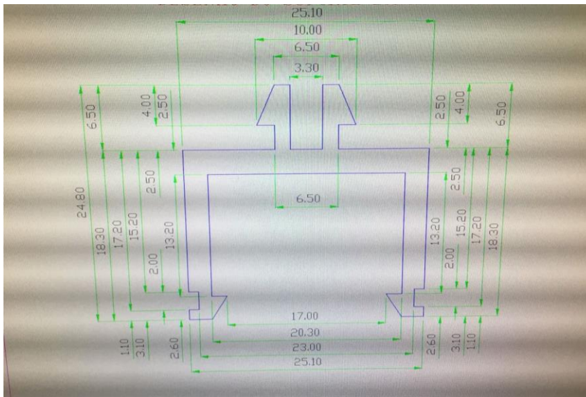
FIGURA 01: DESENHO DA CALHA.
