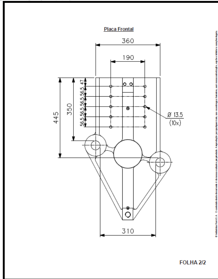
Desenho 02: PLACA FRONTAL DA SOBRADORA
