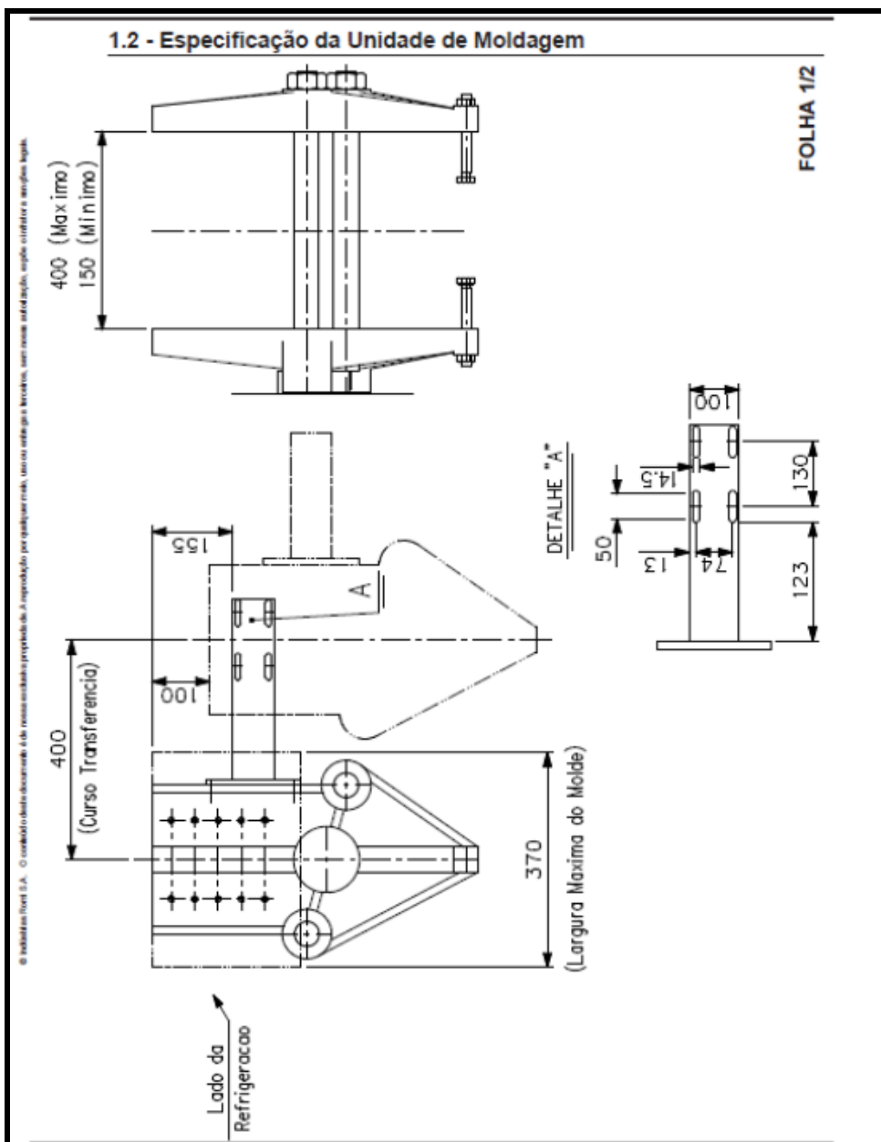
Desenho 01: ESPECIFICAÇÃO DA UNIDADE DE MOLDAGEM SOBRADORA
